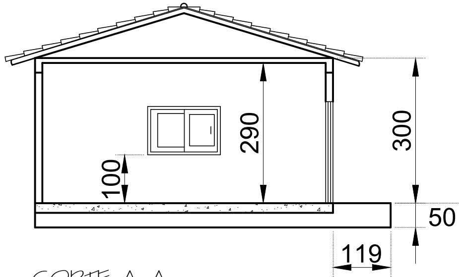
CORTE A-A Escala 1/100
