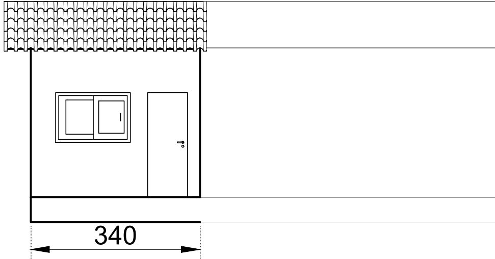
FACHADA Escala 1/100
